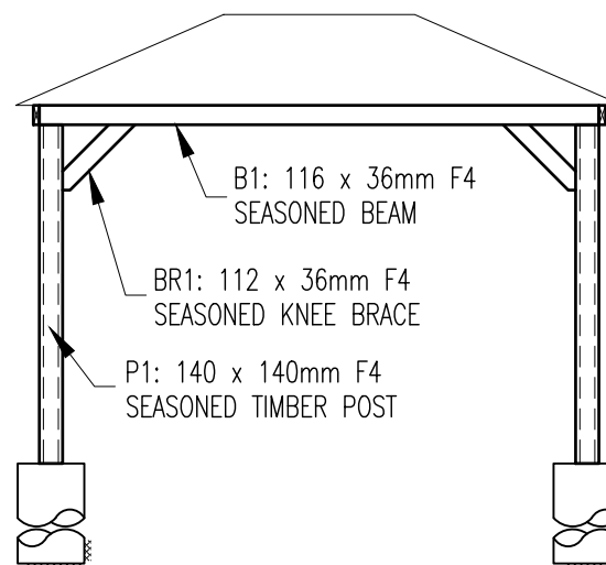
A ELEVATION SCALE: 1:50
