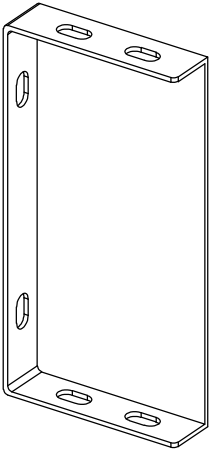
HWH00011 (160*80*22mm)
