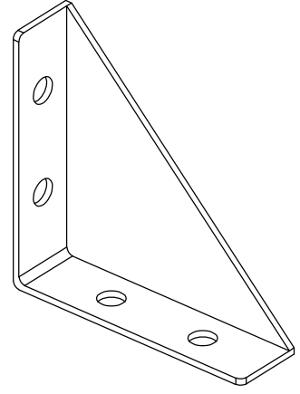
HWH00010 (80*80*22mm)
